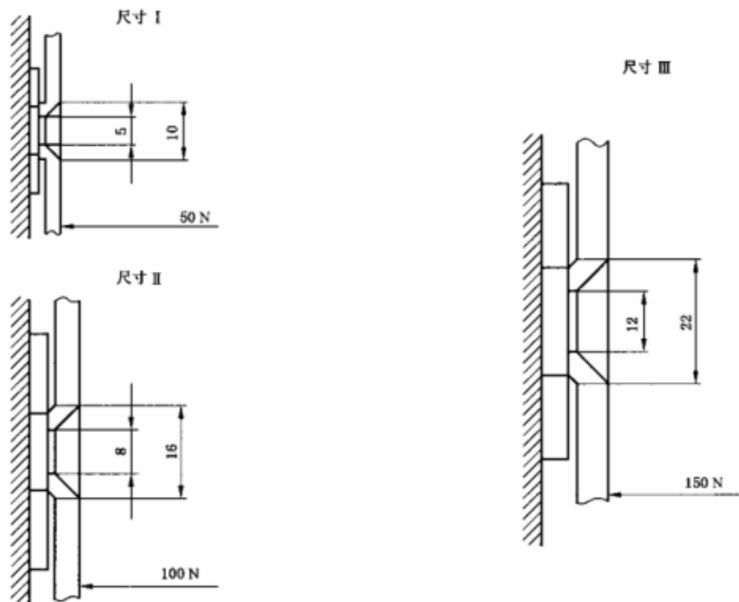
图 A.1 非标准尺寸试样的夹持环
