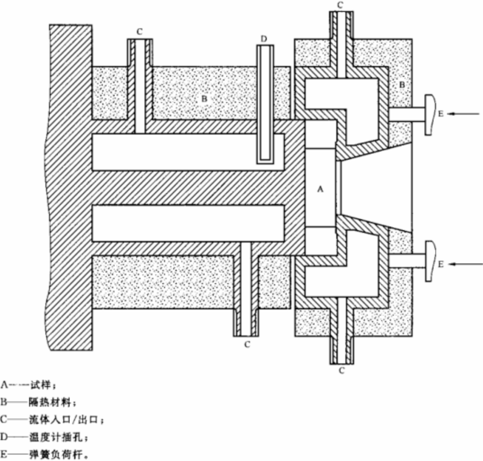
图 3 控温试样夹具示例
